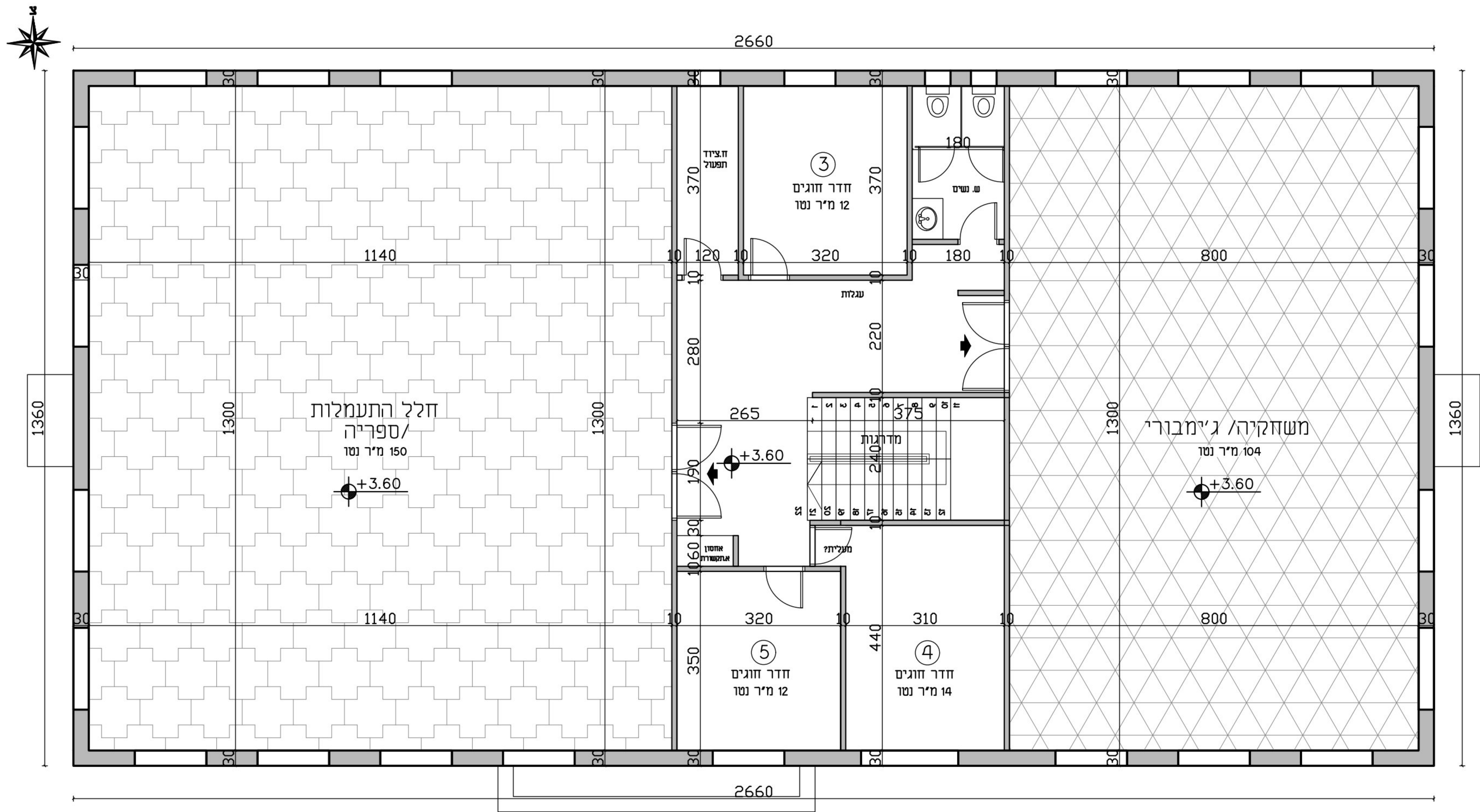
תכנית מפלס עליון מבנה רב תכליתי במפלס זה: 361 מ"ר
