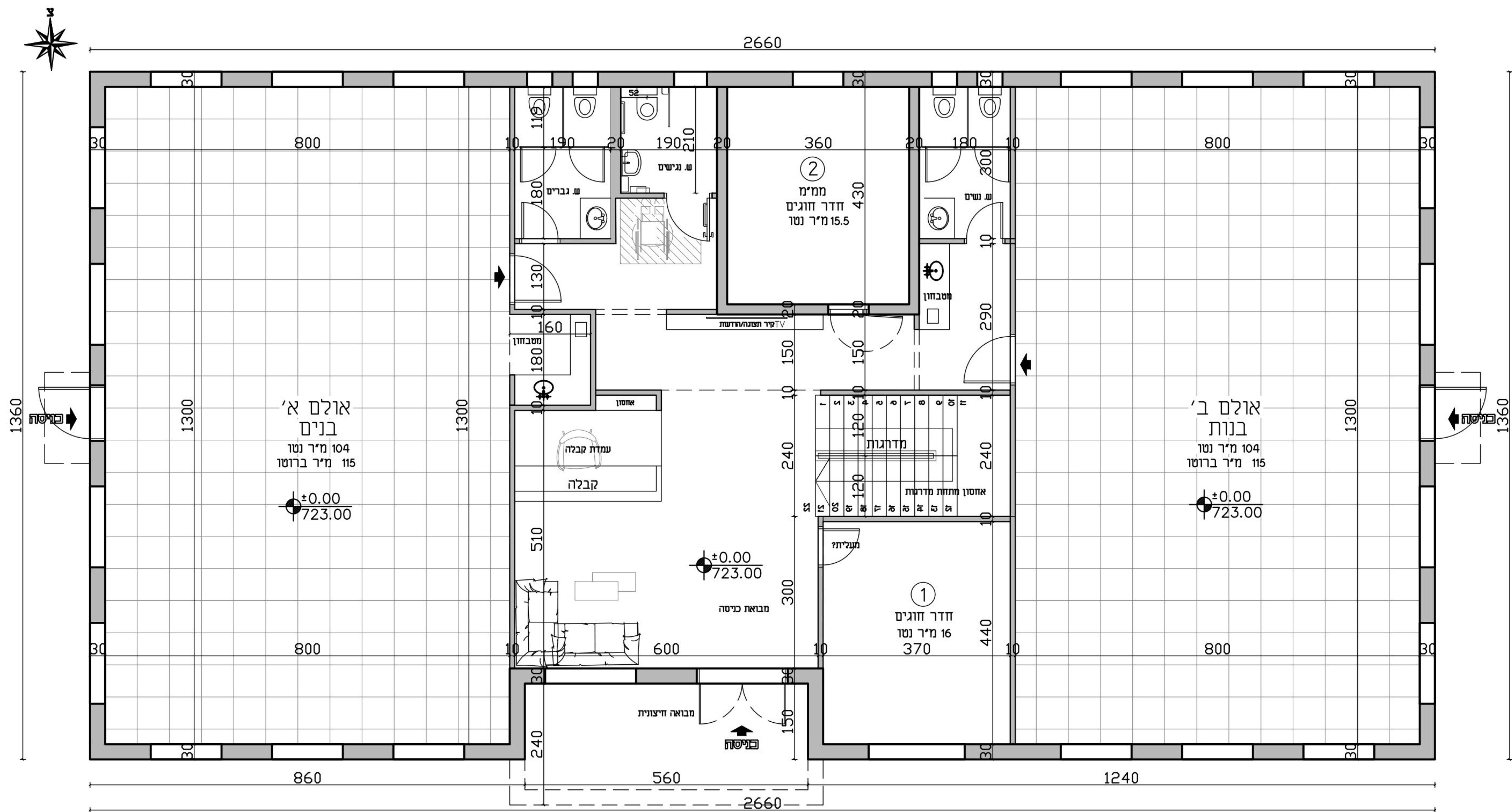
תכנית מפלס בניסה מבנה רב תכליתי במפלס זה: 361 מ"ר
